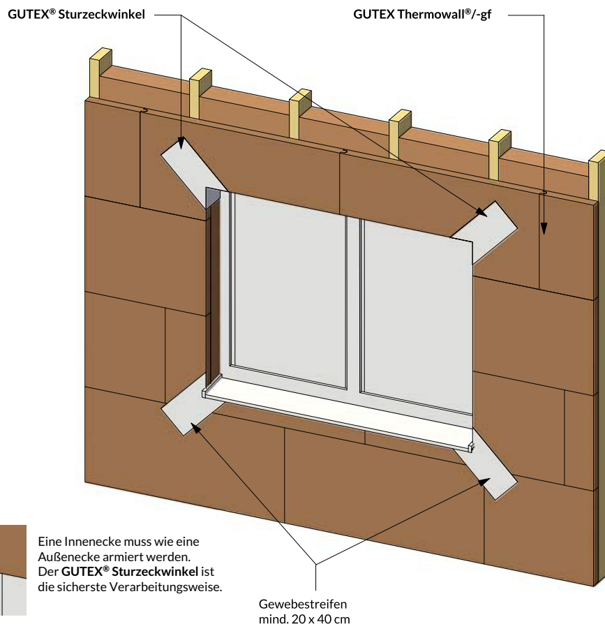
Gebäudeöffnung Diagonalarmierung
